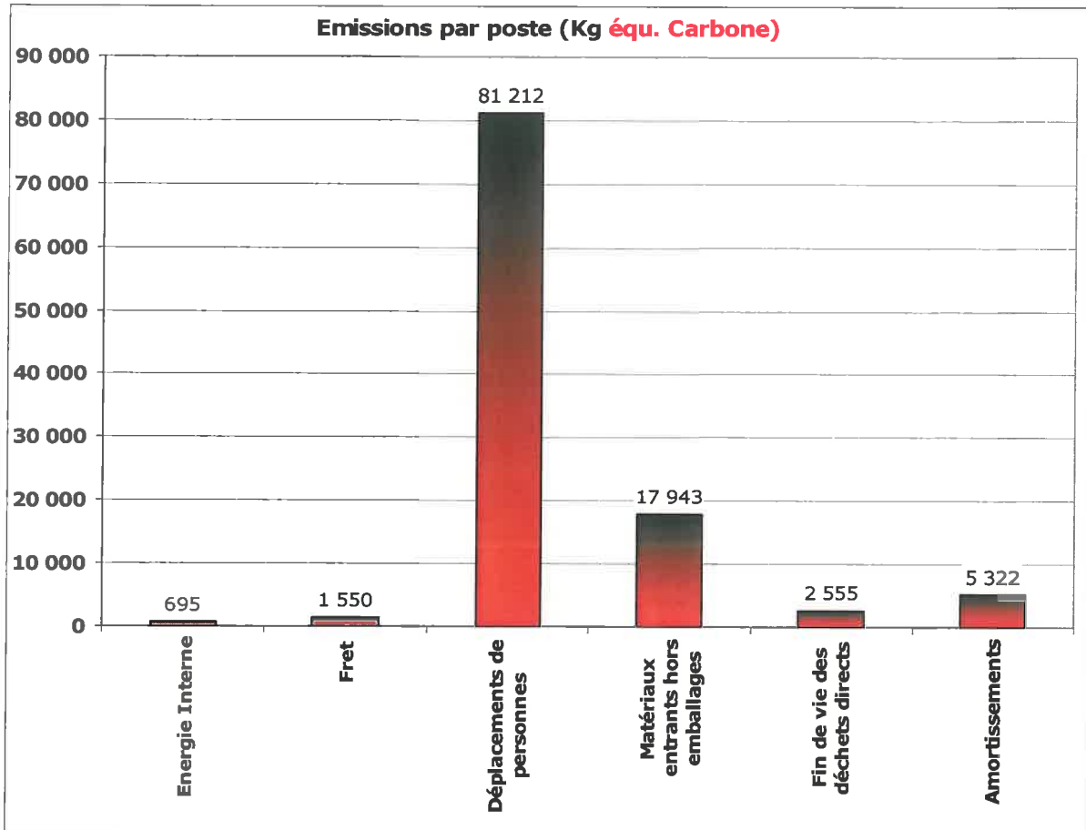
Figure 6 – Synthèse des émissions globale de P.N.S. PrévotEAU
